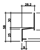
NC-202 水切
