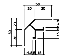
NC-311 入隅
