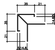
NC-310 出隅
