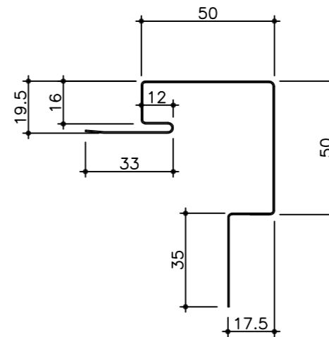
出隅 (K-303)
