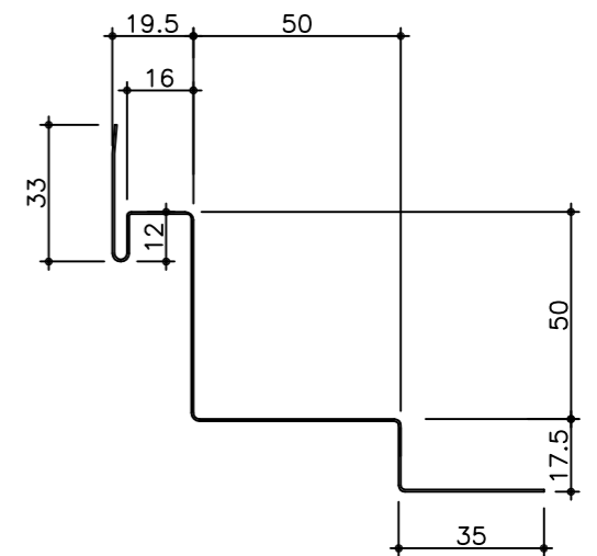
入隅 (K-304)
